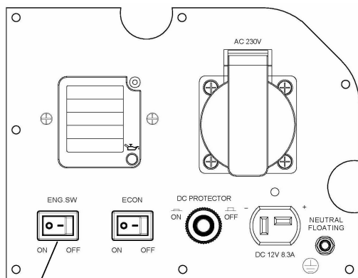
Commutateur de moteur
