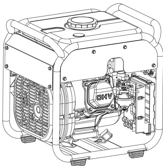
Tiroir de filtre à air
