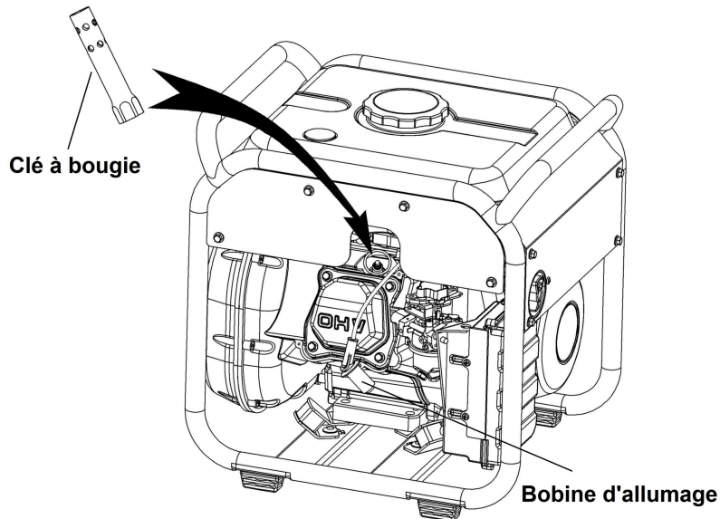
Outil de dépose de bougie
