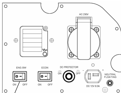
Interrupteur de moteur
