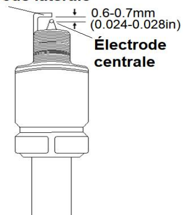
Électrode latérale
